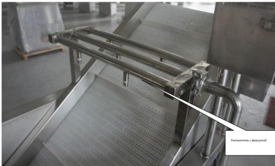
Рис 2. Система очистки, на транспортировочной ленте (форсунки)
